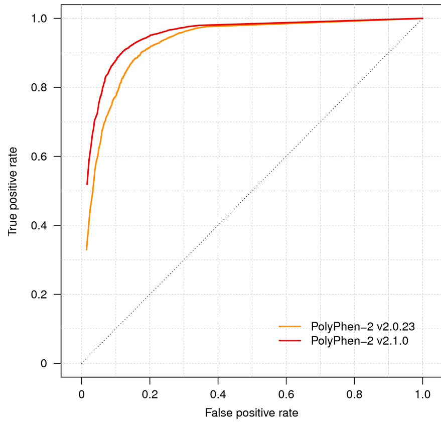
HumDiv / UniRef100
